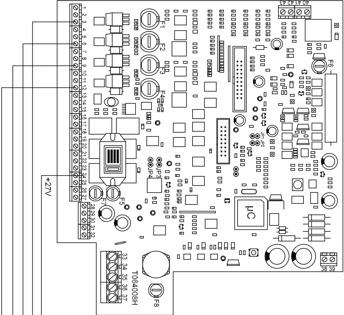
Fig.13: AANSLUTSCHEMA MD644 OPTIONELE RELAISKART 4 RELAIS
