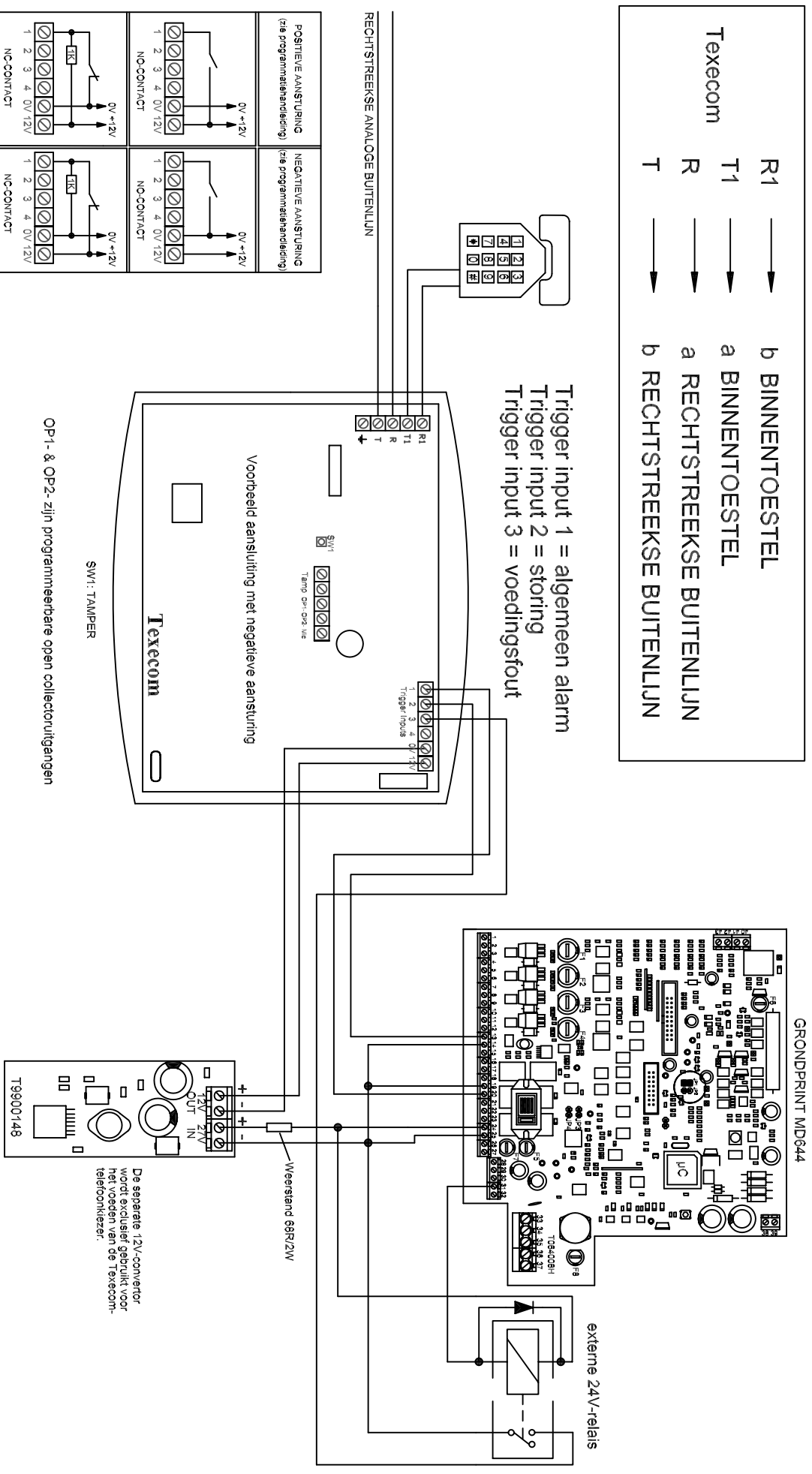
Fig.11: Ansluitschema vocale telefoonkierzer Texecom
