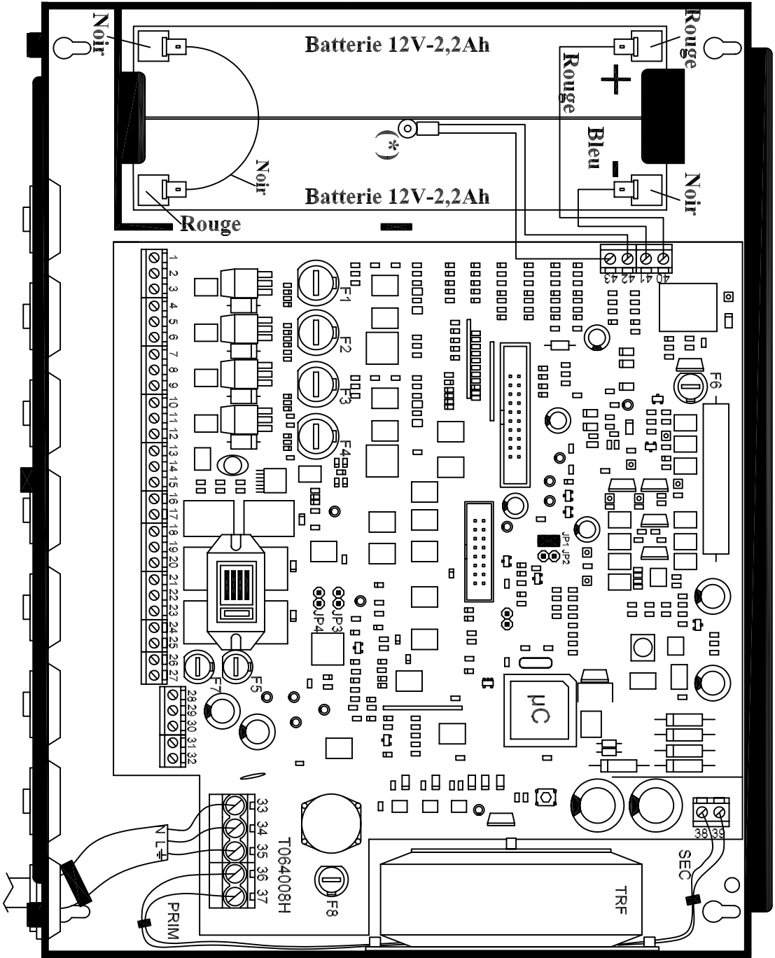
Fig.14: LE BOÎTIER DU CENTRAL MD644
